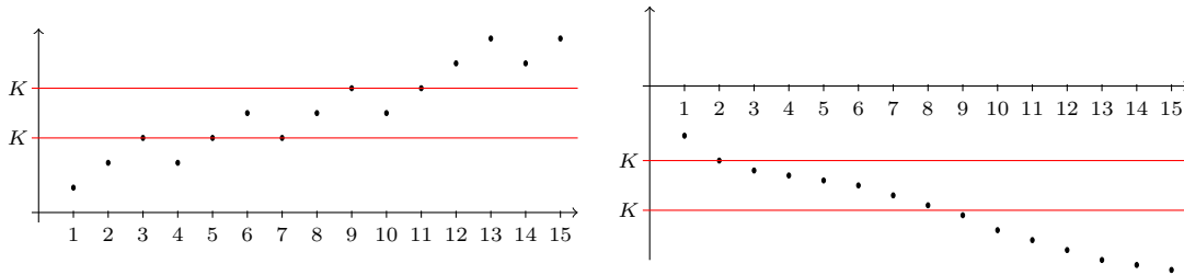
Slika 1.8: Određeno divergentni nizovi.
