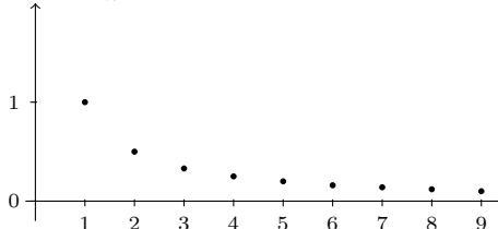
Slika 1.6: Grafički predstavljen niz sa opštim članom x_n = \frac{1}{n} .
