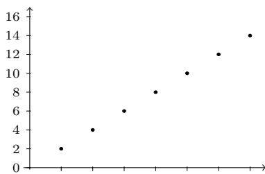
Slika 1.4: Grafički predstavljen niz sa opštim članom x_n = 2n .
