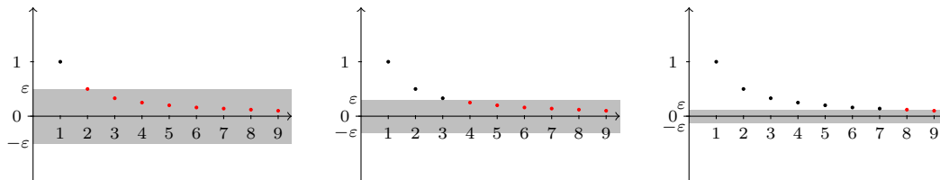
Slika 1.7: Izvan \varepsilon -okoline nalazi se konačno mnogo članova niza.
