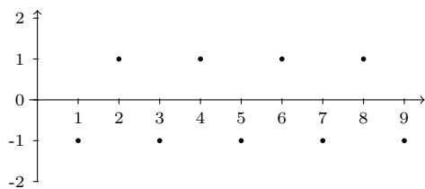
Slika 1.5: Grafički predstavljen niz sa opštim članom x_n = (-1)^n .
